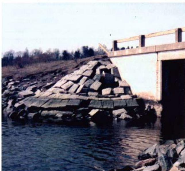
Kuva 1. Kiviheitokkeen eroosioaurion vuoksi sortunut keilaverhous.
